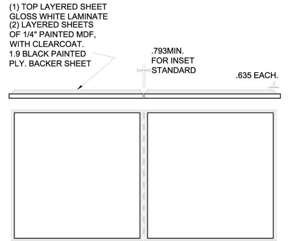
GRID CONSTRUCTION DETAIL SCALE: N.T.S.
