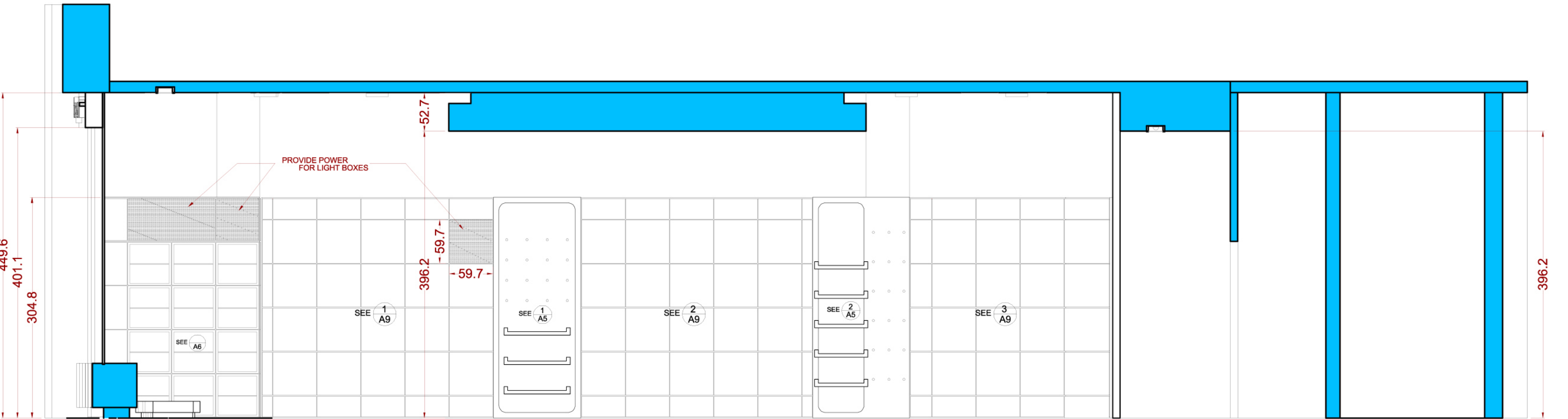
ELEV BB SCALE: 1/4"
